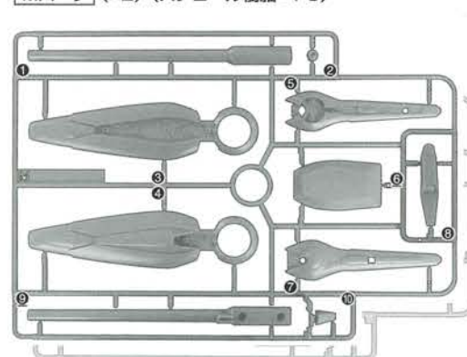
Mパーツ (×2) (スチロール樹脂: PS)
