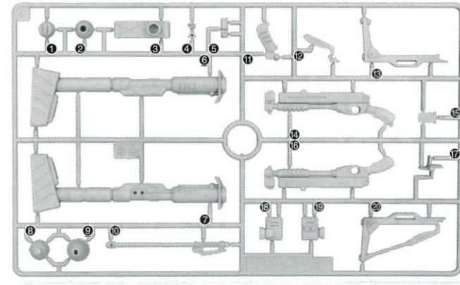
Eパーツ(グレー) (PS) E Parts (Gray)
