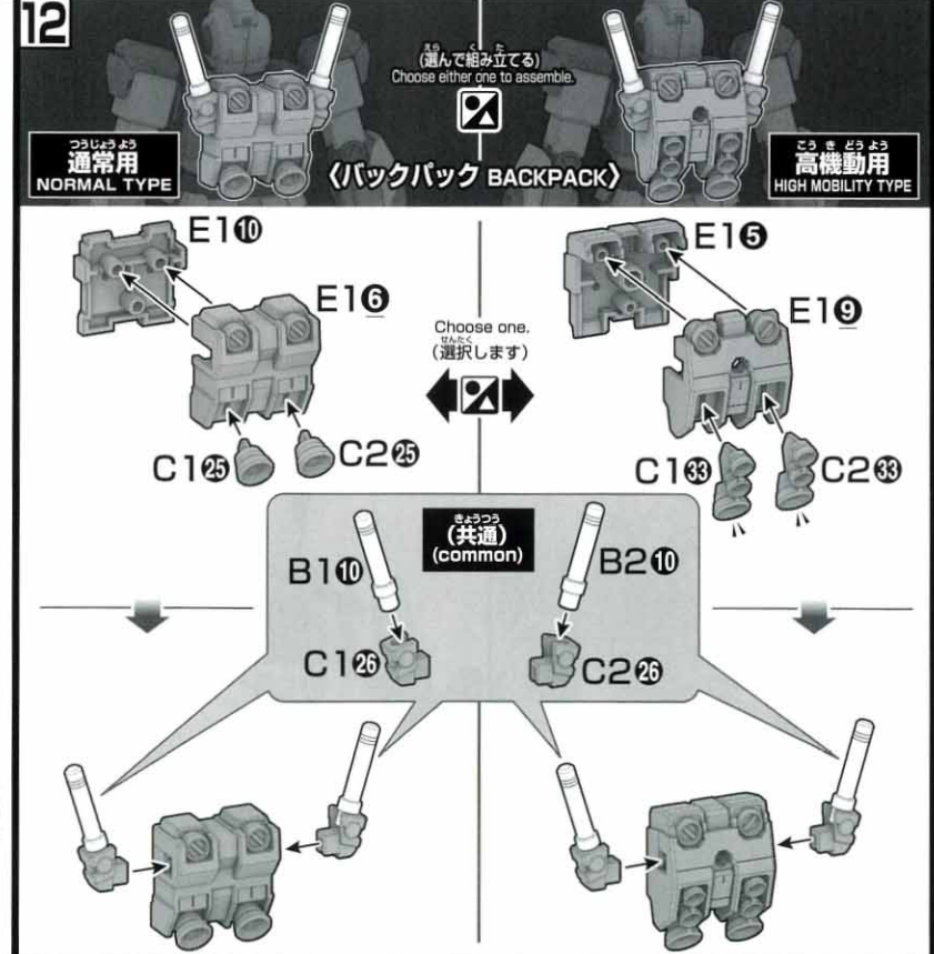
ジーライン・スタンダードアーマー G-LINE STANDARD ARMOR
