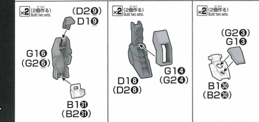
ジーライン・スタンダードアーマー G-LINE STANDARD ARMOR
