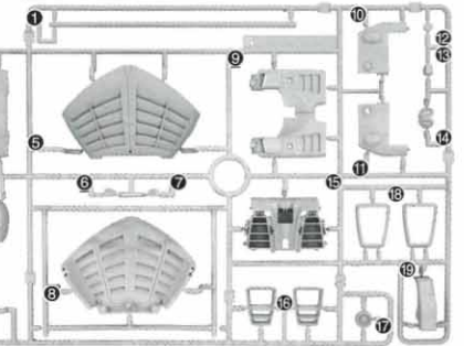
V1パーツ(オレンジ) (PS) V1 Parts (Orange)
