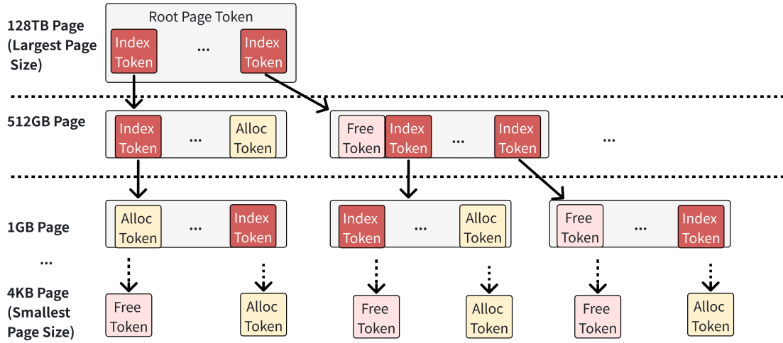
图 4-2 PageAllocator 结构
