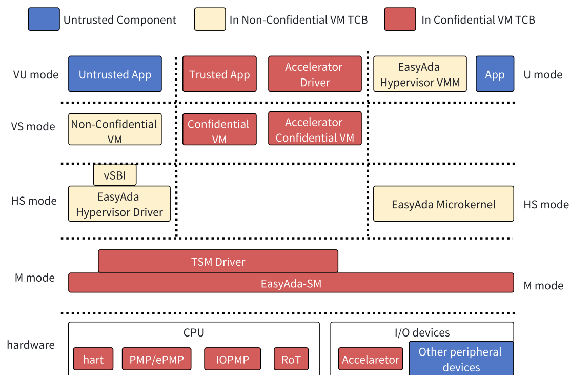
图 3-1 基于 RISC-V 的微内核虚拟化方案总体架构
