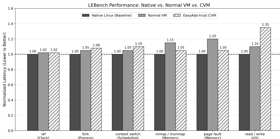
图 6-8 LEBench 测试结果
