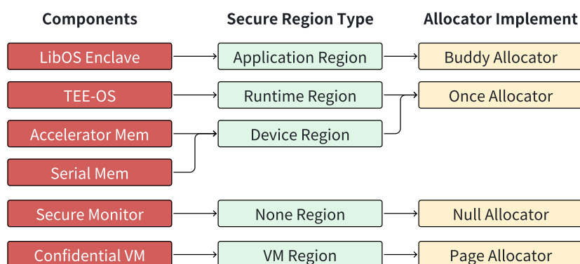
图 4-6 不同类型飞地与区域类型和分配器的关联关系
