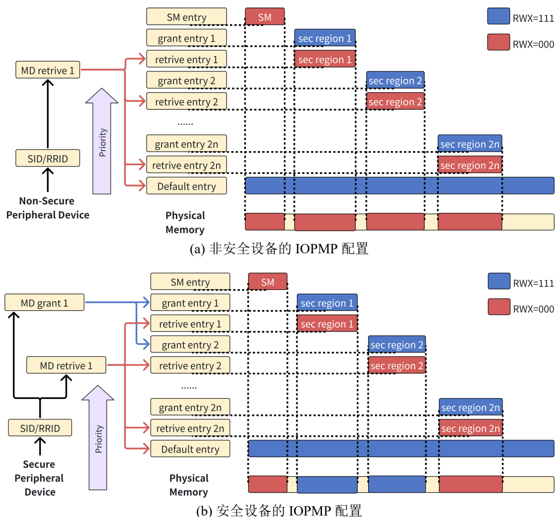
图 4-8 EasyAda -安全监视器中非安全/安全设备的 IOPMP 管理
