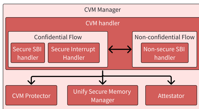
图 4-7 机密虚拟机管理器结构
