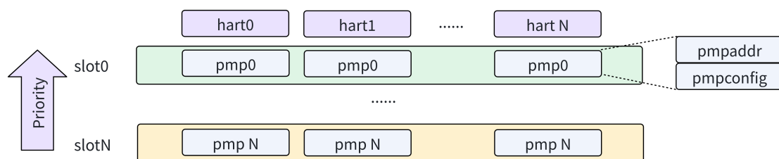
图 4-3 PMP 槽结构
