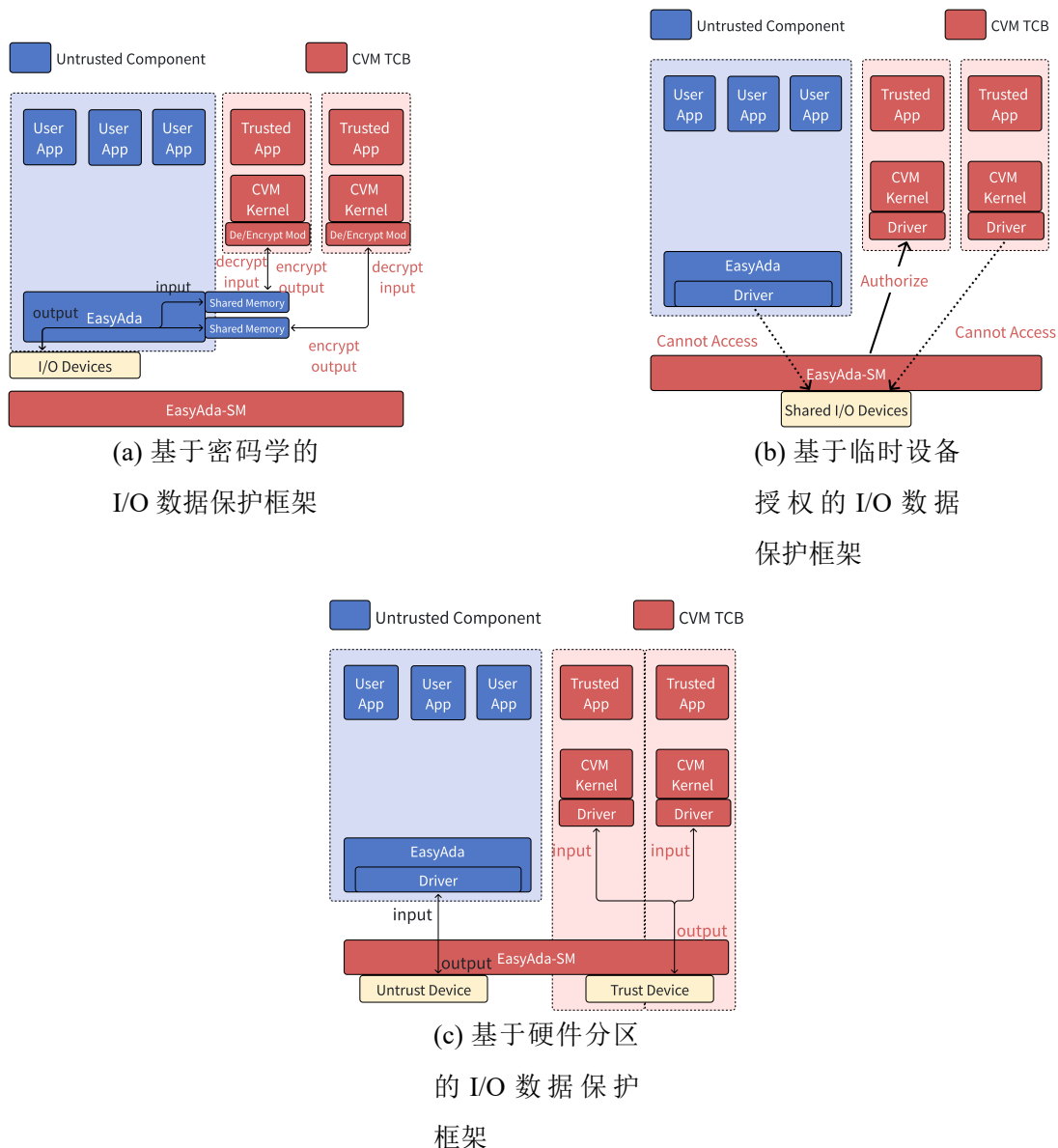
图 3-6 CVM 的 I/O 数据保护机制
