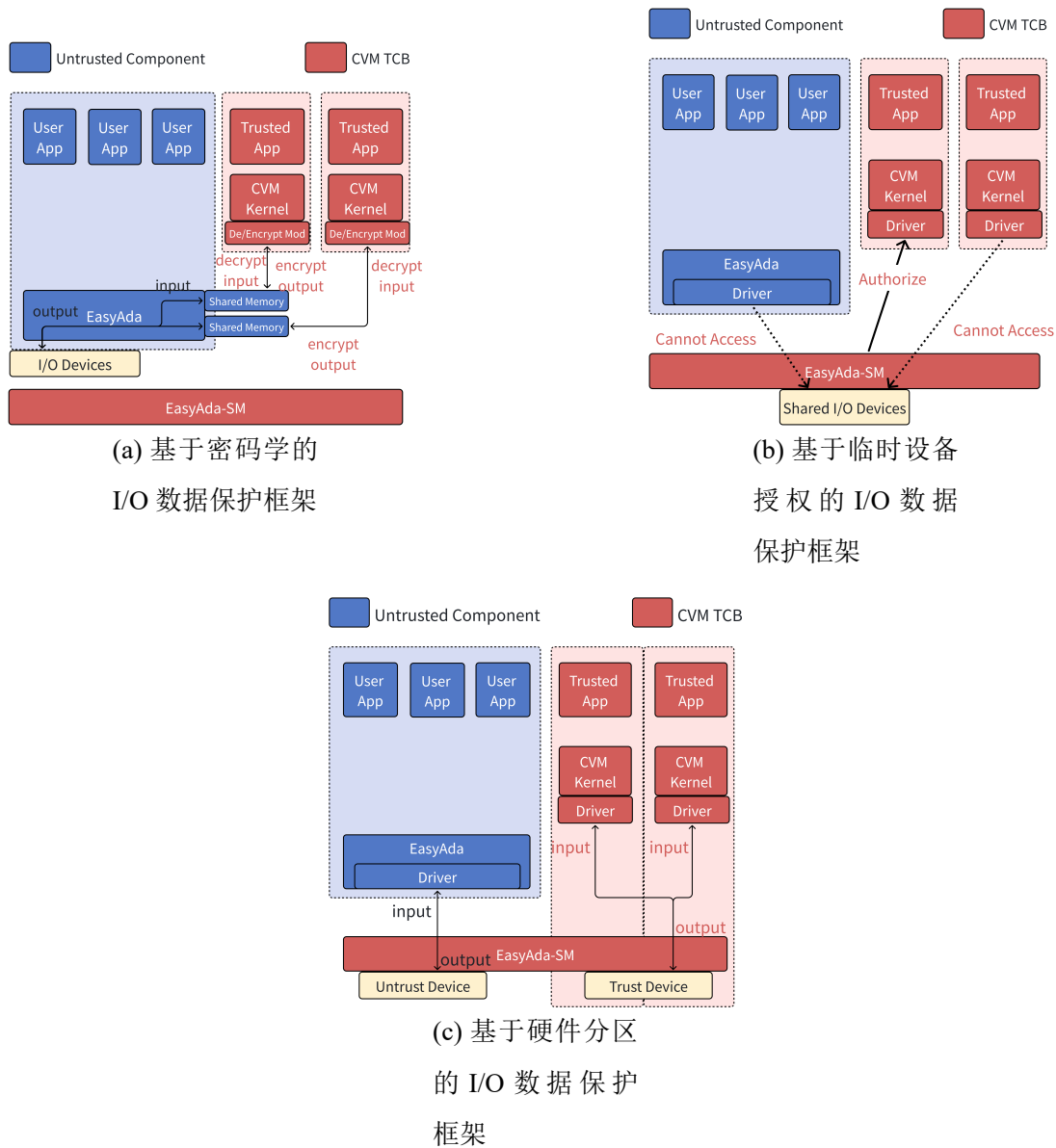
图 3-7 CVM 的 I/O 数据保护机制
