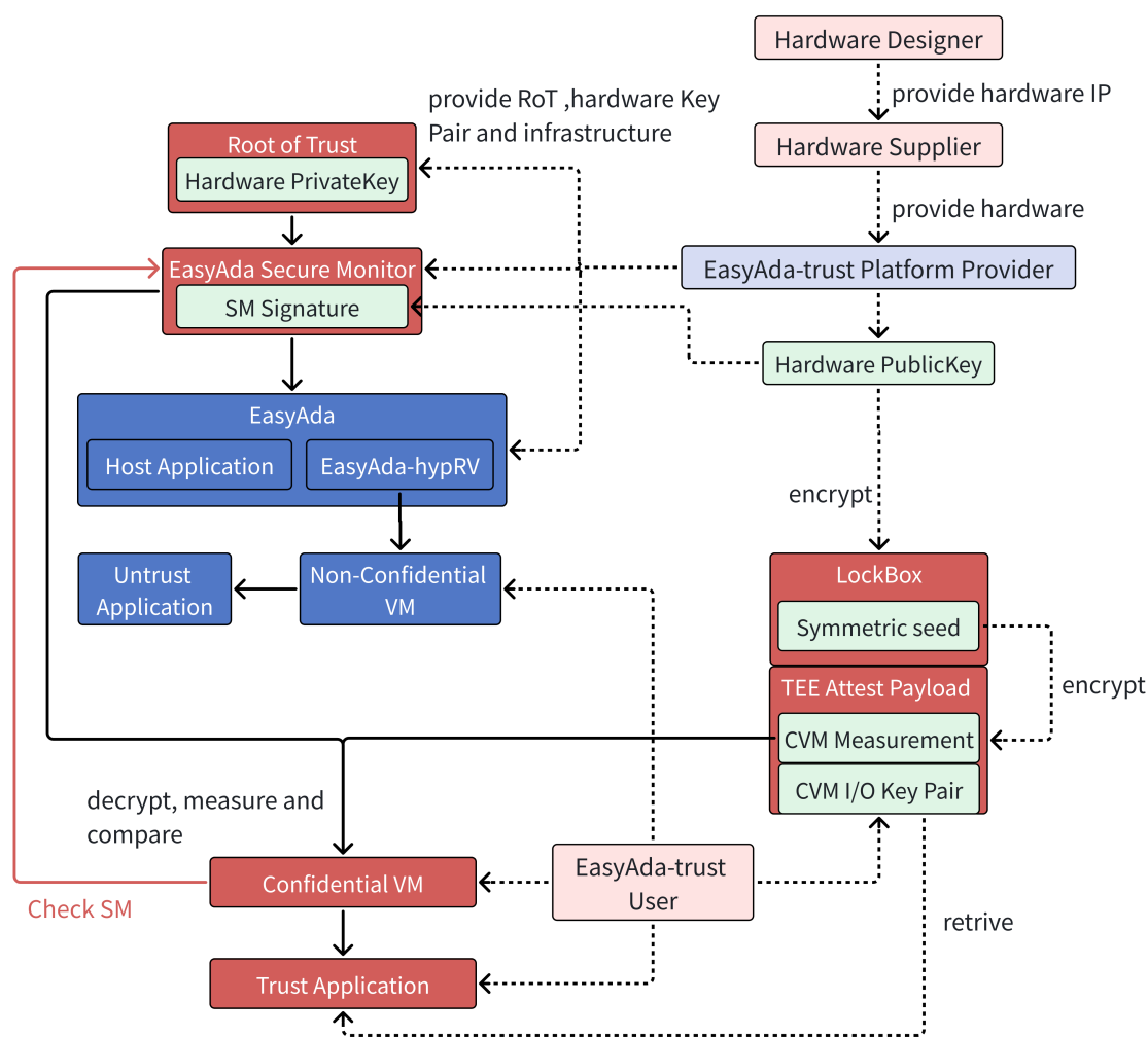
图 3-5 EasyAda-trust 可信启动流程
