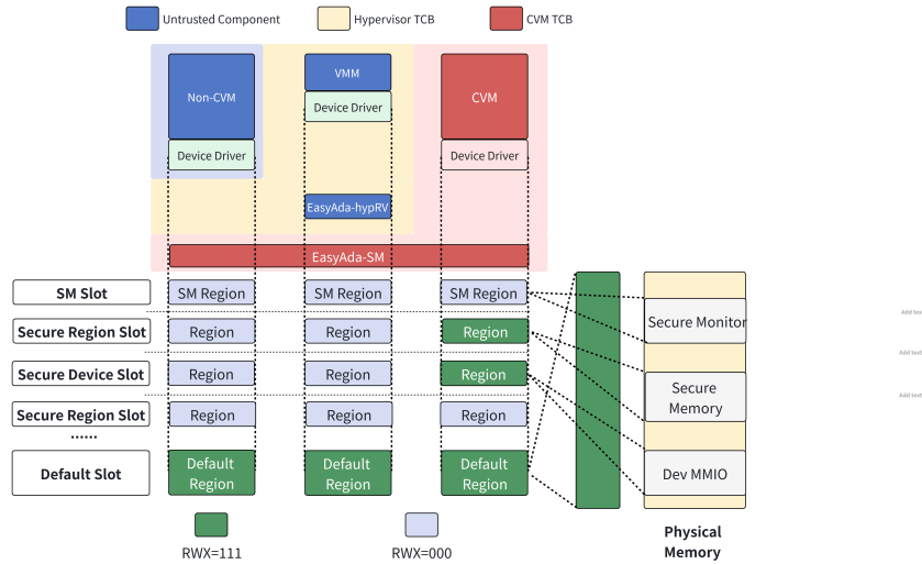
图 5-3 引入安全设备后的 CVM 安全内存视图
