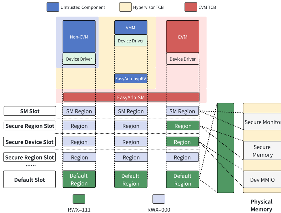
图 5-6 引入安全设备后的 CVM 安全内存视图
