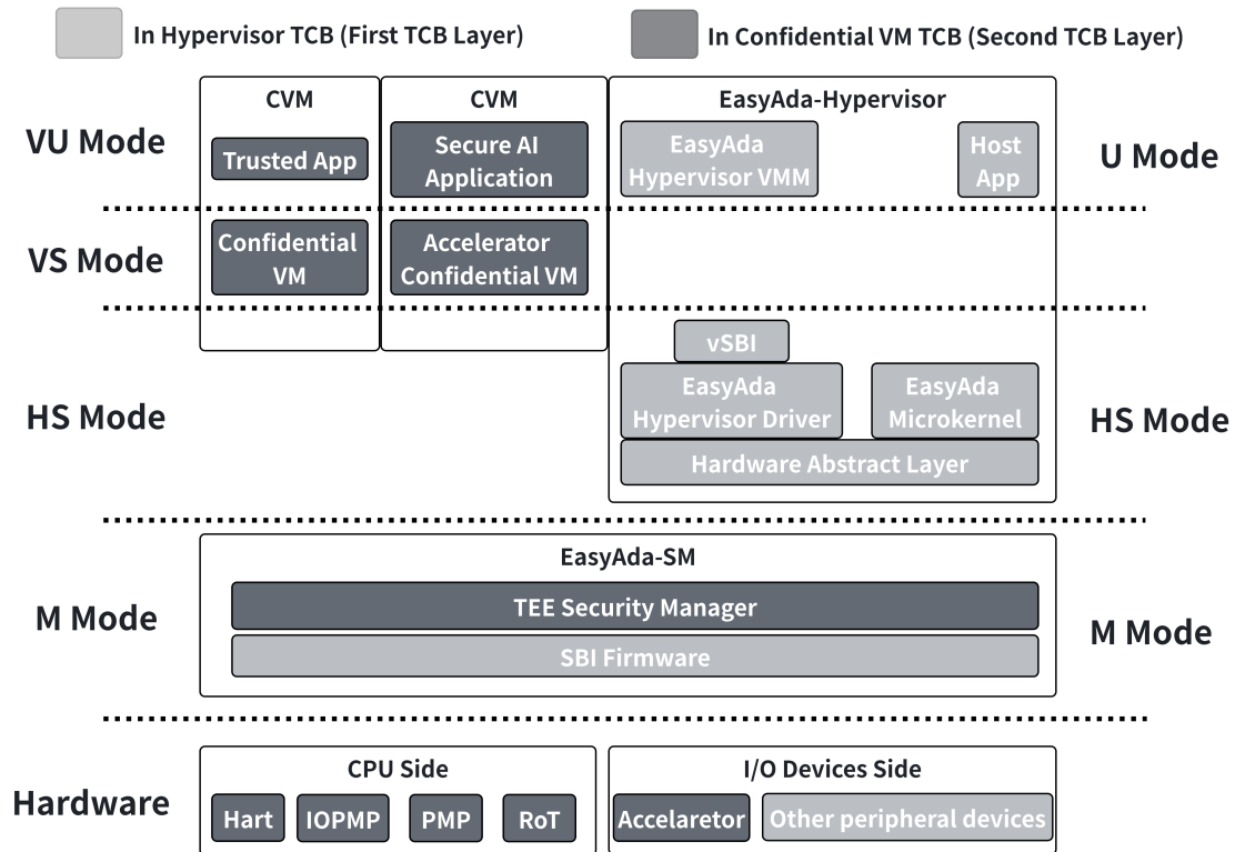
图 3-2 机密虚拟机可信基
