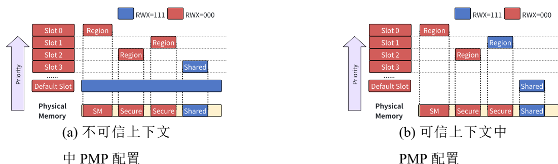
图 4-4 PMP 运行时配置
