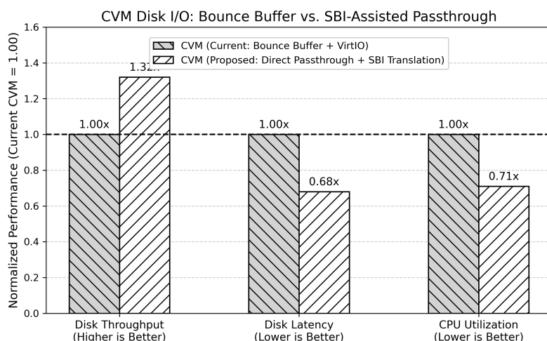
图 6-9 安全设备直通架构与半虚拟化机制（不可信共享内存）下的磁盘 I/O 对比测试结果
