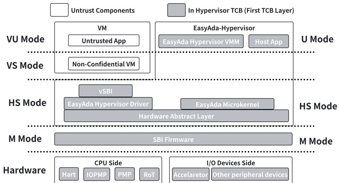
图 3-1 非机密虚拟机可信基
