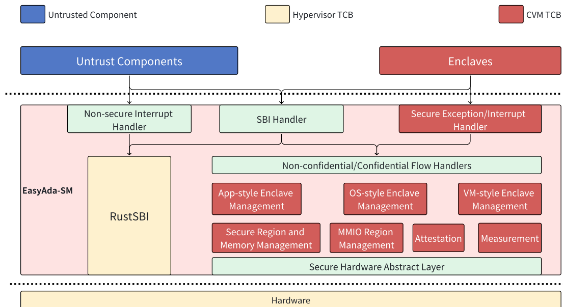
图 3-4 EasyAda-SM 总体架构
