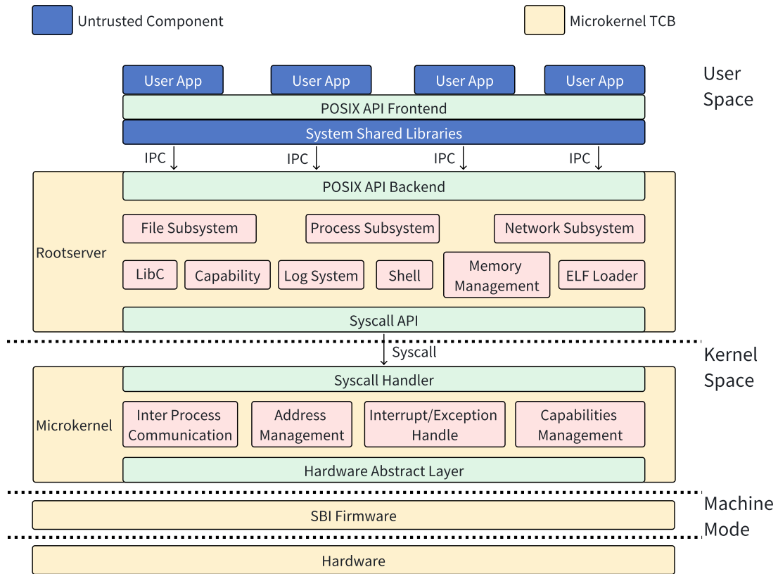
图 3-1 微内核操作系统 EasyAda 总体架构
