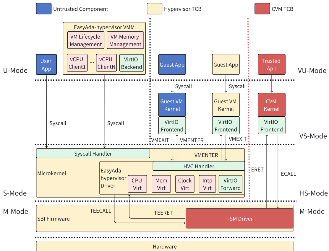
图 3-2 EasyAda-hypervisor 总体架构
