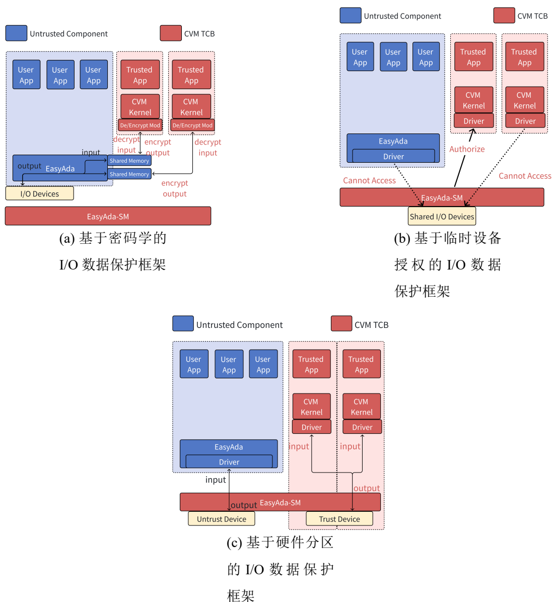
图 3-8 CVM 的 I/O 数据保护机制
