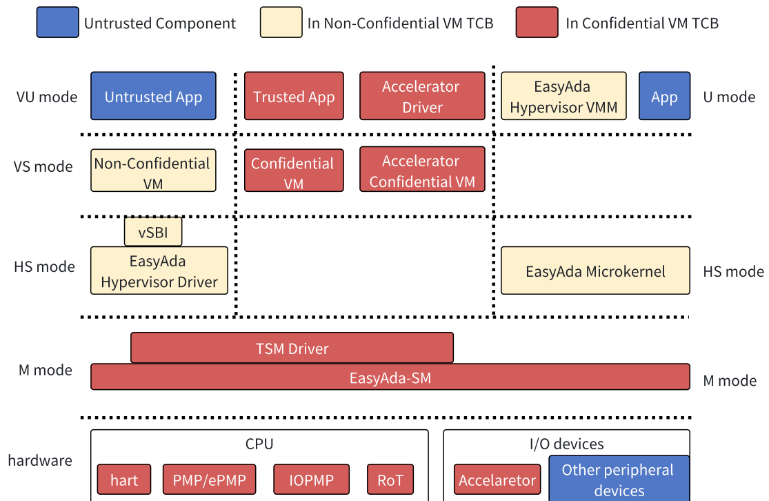
图 3-3 基于 RISC-V 的微内核虚拟化方案总体架构
