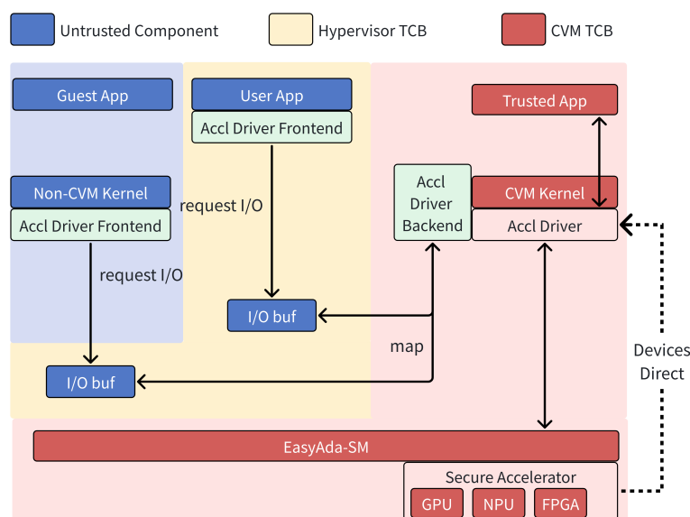
图 3-9 硬件加速器管理 CVM 设计
