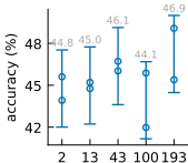
HCP-A Age
