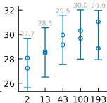
NSD COCO24
