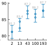
HCP-A Sex
