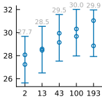
NSD COCO24
