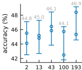
HCP-A Age
