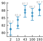
HCP-A Sex
