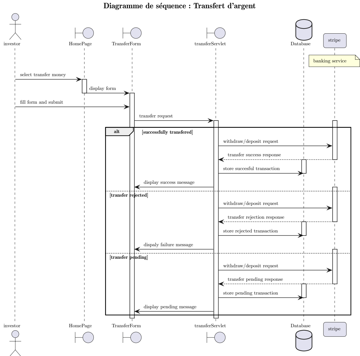
FIGURE 3 – Diagramme de séquence : Transfert d'argent
