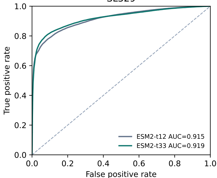
SL329
