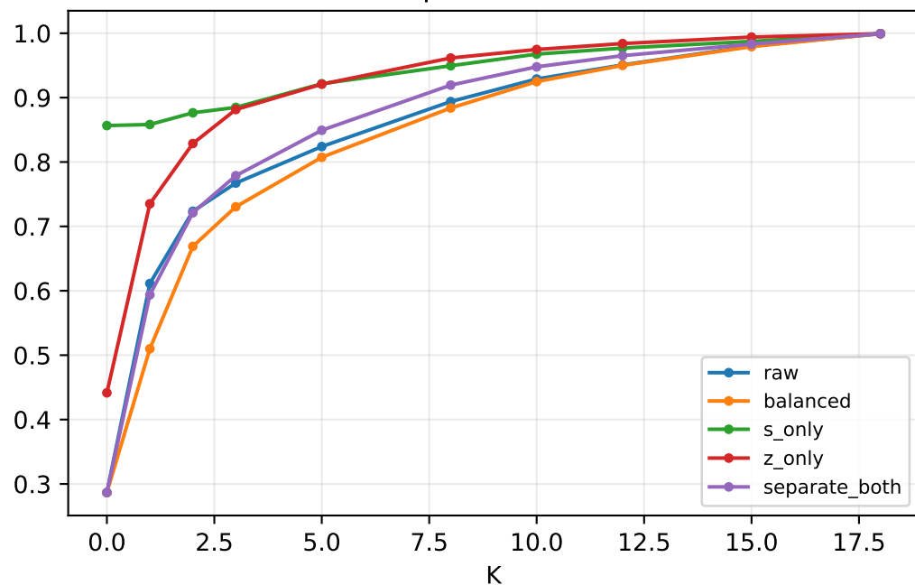
Local RMSD > 1 Å / 1900
