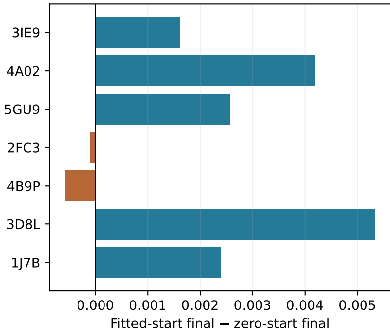
All-atom IDDT
