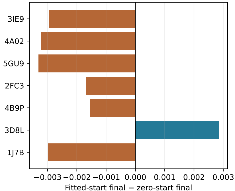
Cα-IDDT
