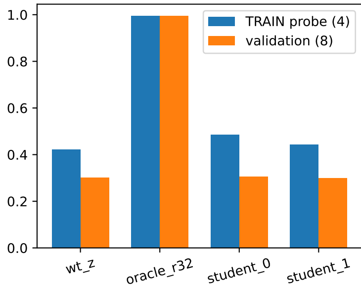
19-AA Spearman
