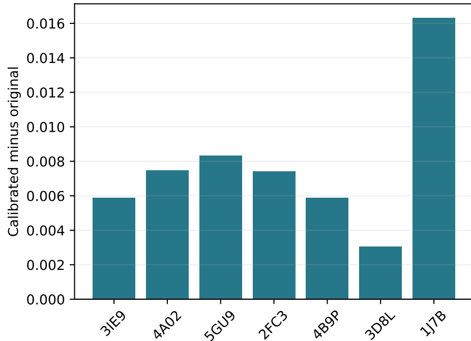
All-atom IDDT
