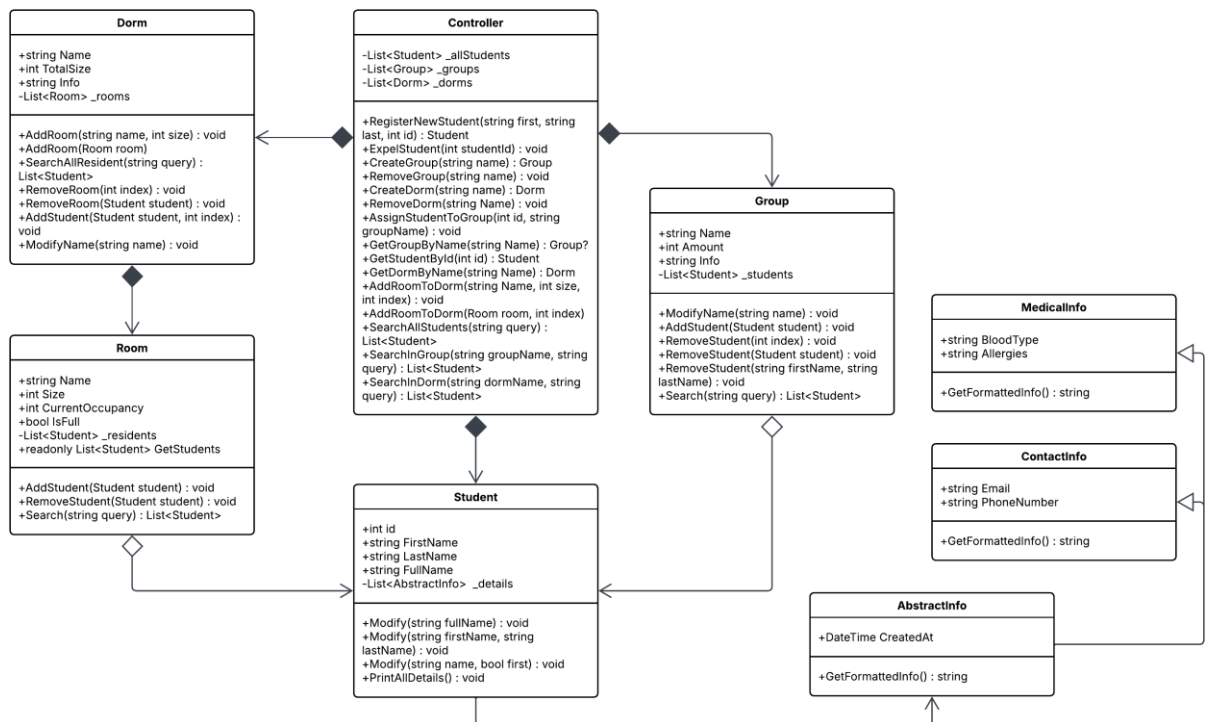
Рис. 1. Діаграма класів
