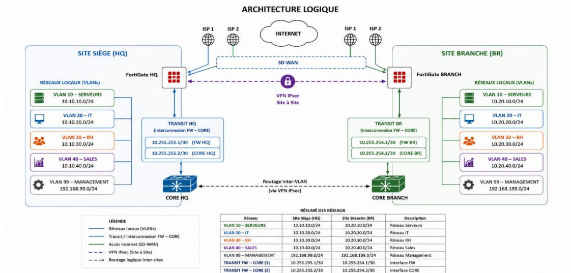
Figure 2 — Topologie logique du réseau HQ et BR
