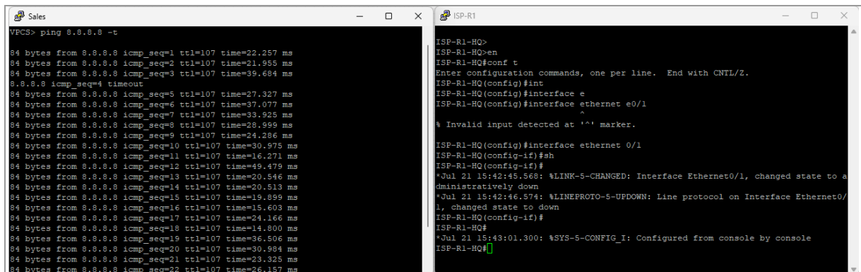
Figure 25 — Résultat du test — Basculement ISP1 → ISP2
