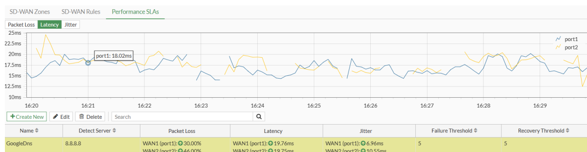
Figure 22 — Résultat du test — Dashboard SD-WAN
