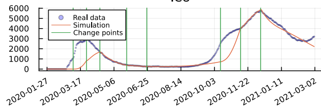
ICU
