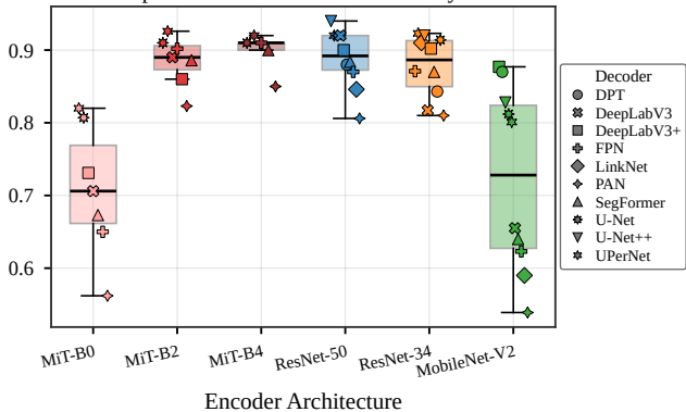
Impact of Encoder on Test Boundary F1
