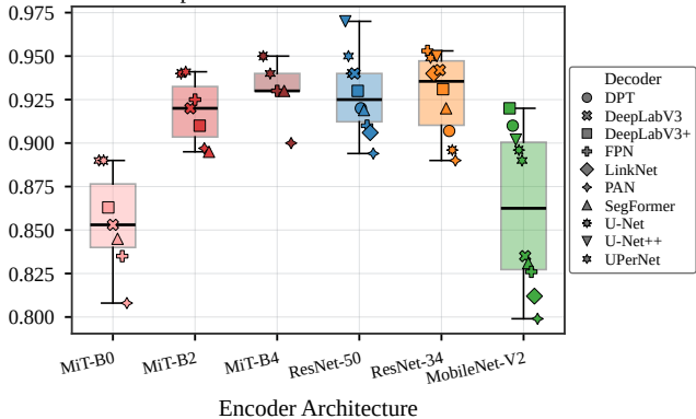
Impact of Encoder on Test Dice F1
