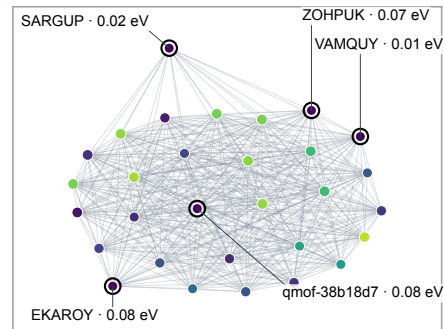
e Low-gap region (O2 hits)
