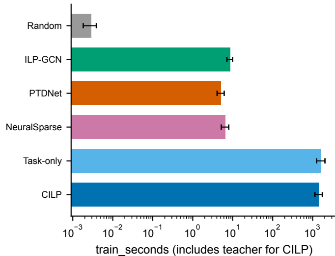
Facebook Page-Page (CPU)
