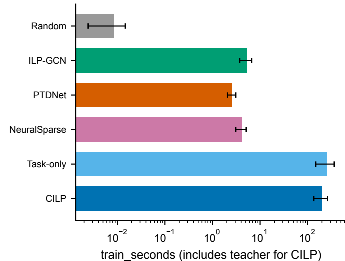
LastFM Asia (CPU)
