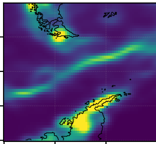
(f) Replicate-fill
