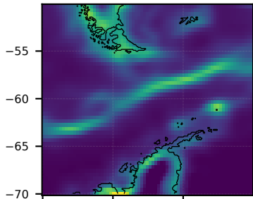
(f) Zero-fill
