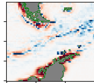
(f) Replicate-fill
