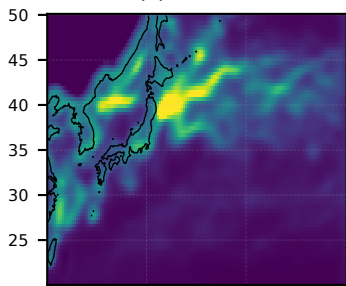
(f) Zero-fill
