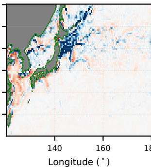
(f) Replicate-fill
