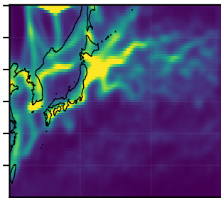
(f) Replicate-fill
