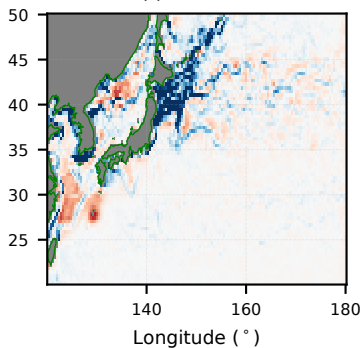
(f) Zero-fill
