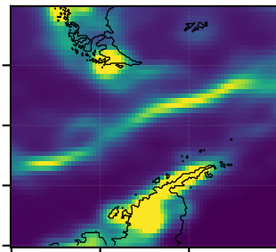
(f) Replicate-fill
