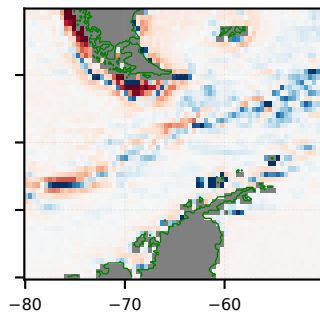
(f) Laplace-fill
