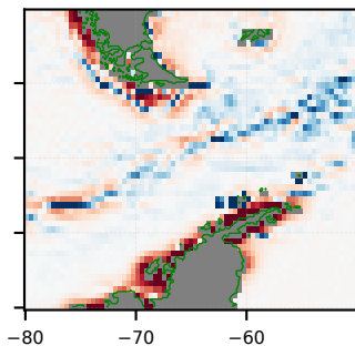
(f) Replicate-fill
