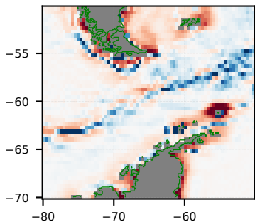
(f) Zero-fill
