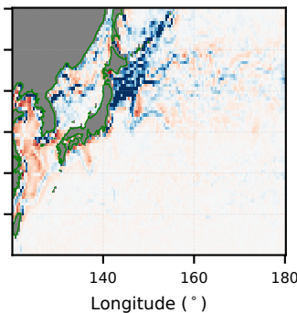
(f) Replicate-fill
