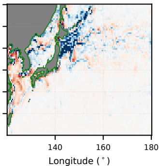
(f) Laplace-fill
