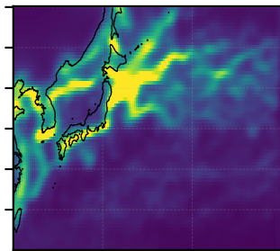
(f) Laplace-fill
