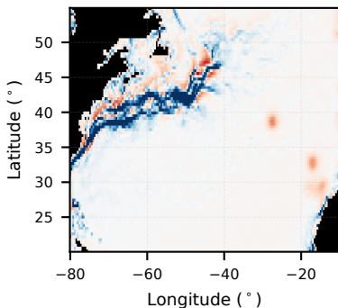
(d) Zero-fill
