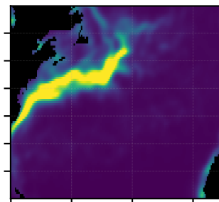
(f) Laplace-fill
