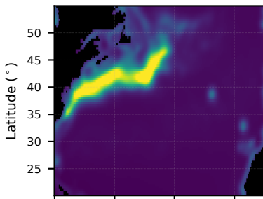
(d) Zero-fill
