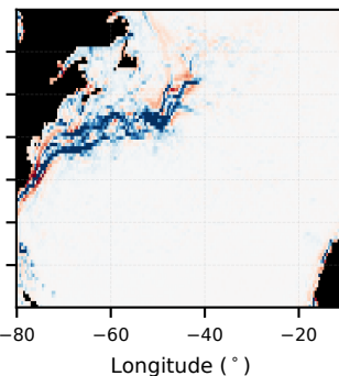
(f) Laplace-fill
