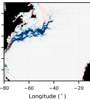
(e) Replicate-fill
