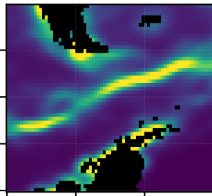
(e) Replicate-fill
