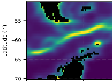
(d) Zero-fill
