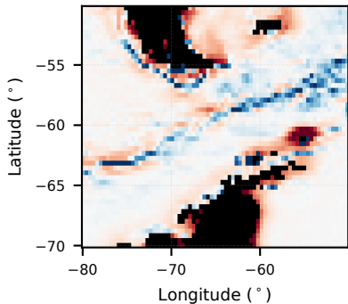
(d) Zero-fill
