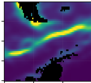
(f) Laplace-fill
