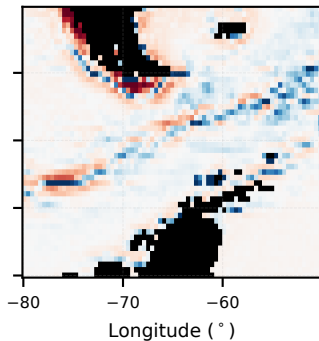
(f) Laplace-fill
