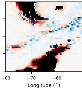
(e) Replicate-fill
