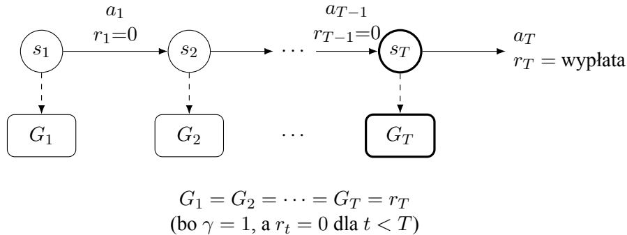
Rys. 5.7. Zwrot G_t w epizodzie REINFORCE
