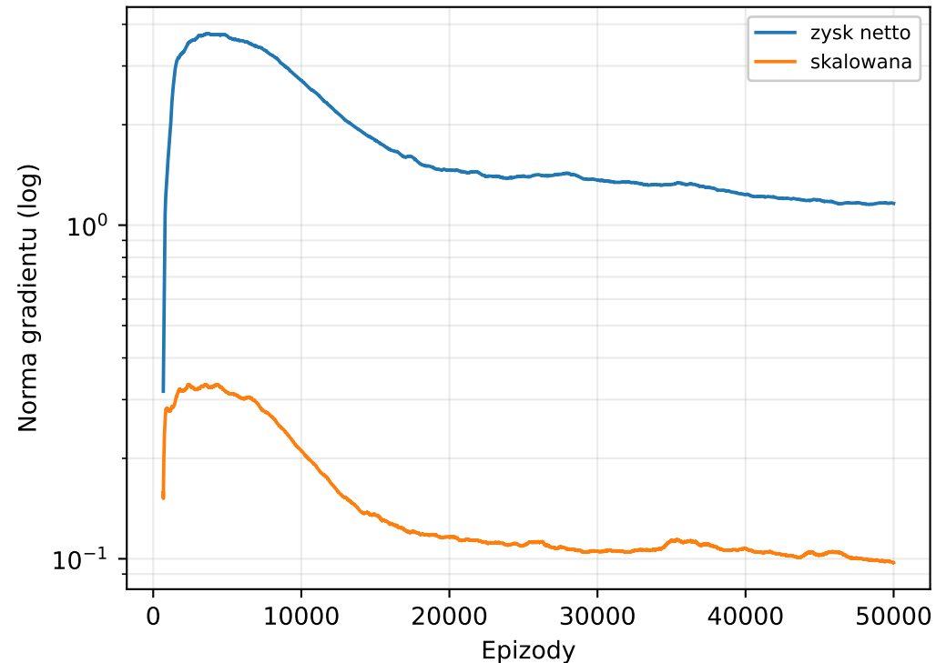
DQN
