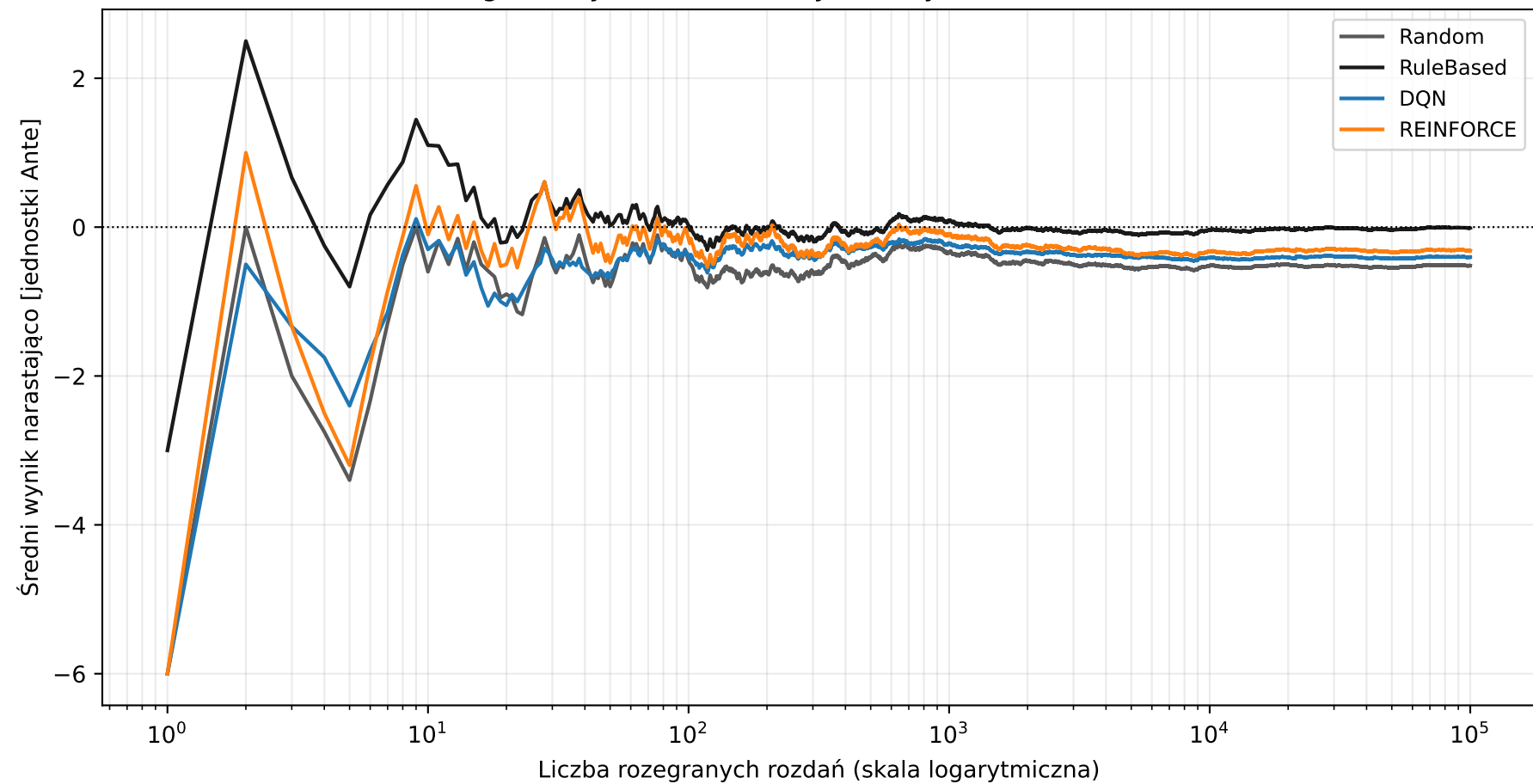
Zbieganie wyniku do EV na tym samym rozkładzie rozdań
