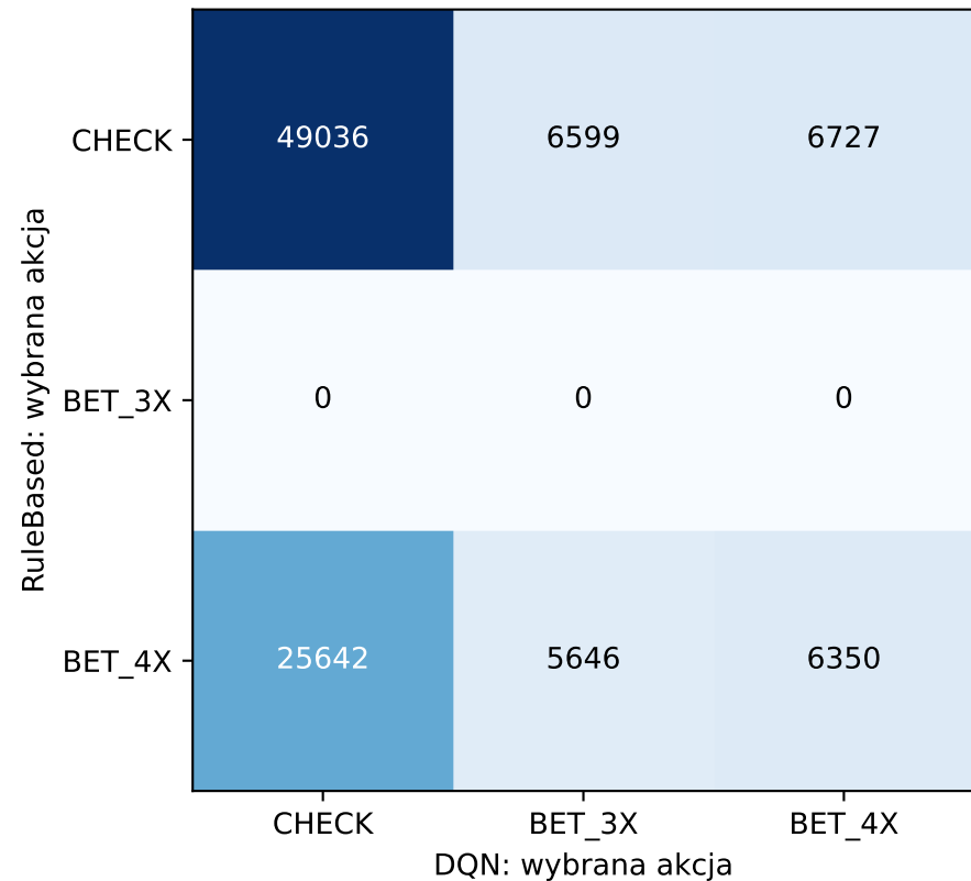
DQN vs RuleBased (zgodność 55.4%)
