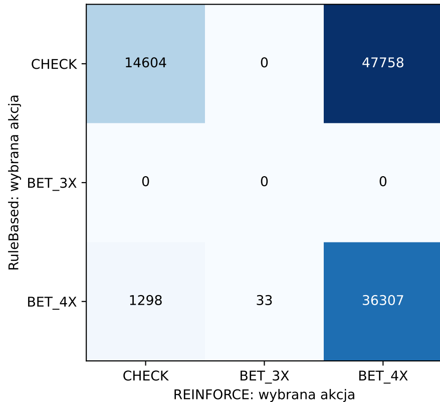
REINFORCE vs RuleBased (zgodność 50.9%)
