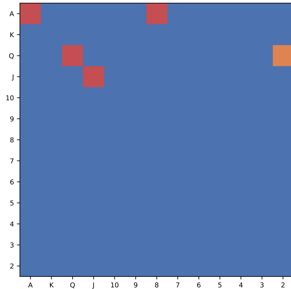
DQN
