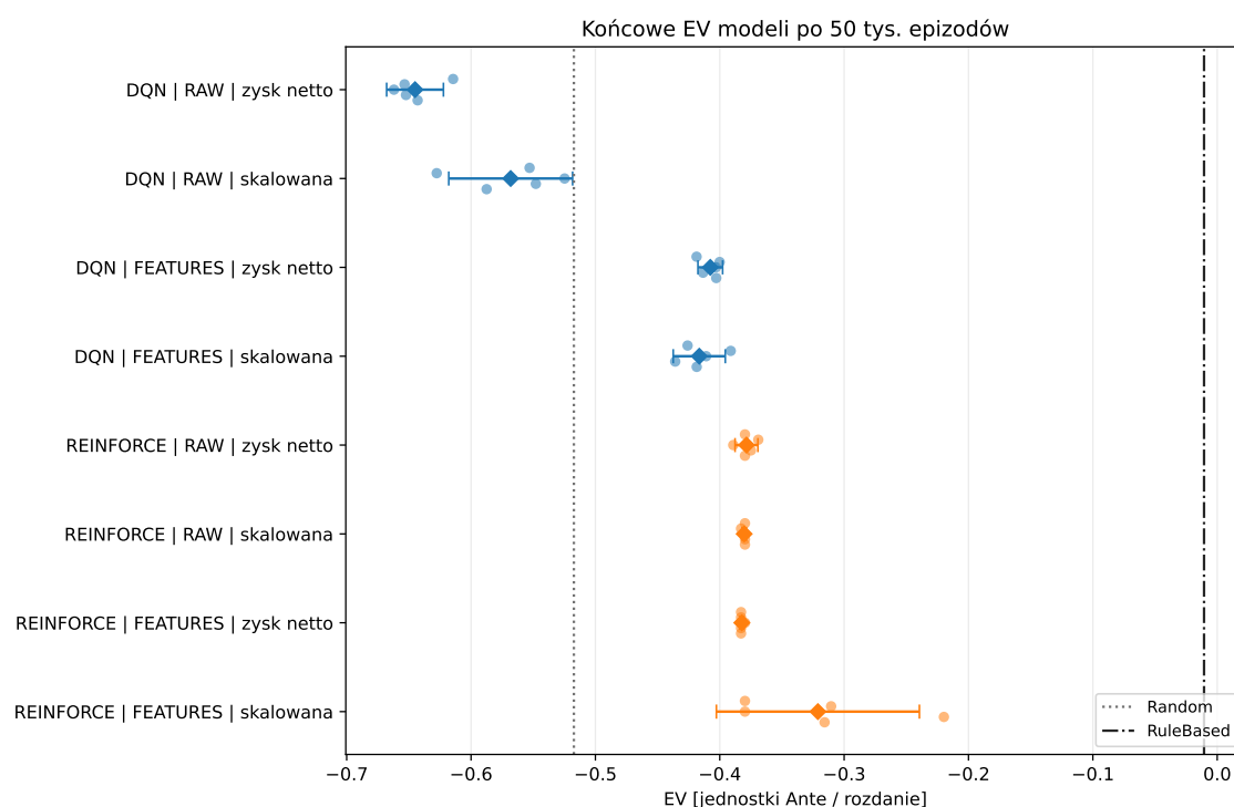
Rys. 7.1. Końcowe wartości EV ośmiu konfiguracji po 50 000 epizodów treningowych. Małe punkty przedstawiają wyniki poszczególnych seedów, a większe znaczniki średnie wartości konfiguracji wraz z 95-procentowymi przedziałami ufności wyznaczonymi na podstawie pięciu przebiegów treningowych. Linie pionowe oznaczają wyniki agentów Random i RuleBased.
