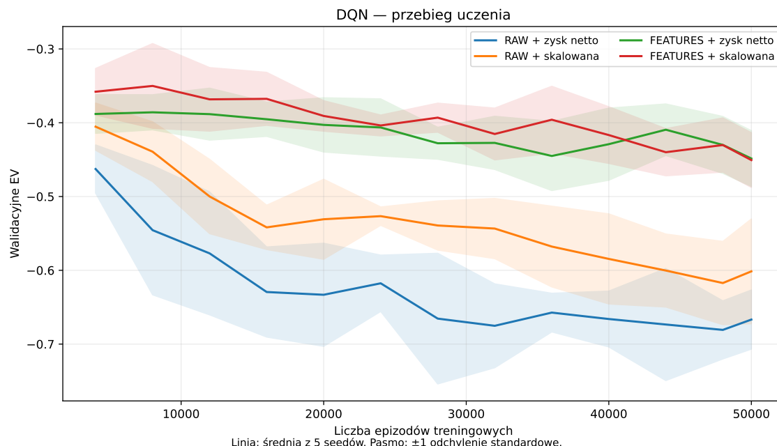
Rys. 7.4. Przebieg uczenia czterech konfiguracji DQN. Linie przedstawiają średnie walidacyjne EV z pięciu seedów, natomiast pasma odpowiadają jednemu odchyleniu standardowemu między przebiegami treningowymi.
