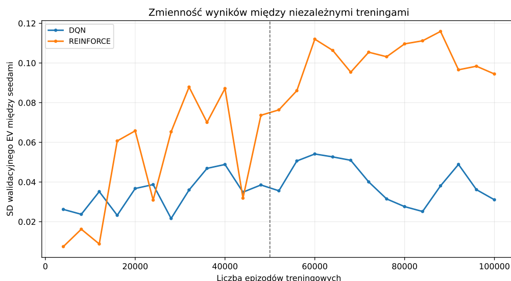
Rys. 7.7. Zmienność walidacyjnego EV pomiędzy pięcioma seedami podczas treningu wybranych konfiguracji DQN i REINFORCE. Oś pionowa przedstawia odchylenie standardowe wartości EV między przebiegami treningowymi.
