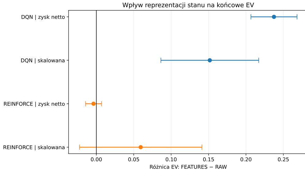
Rys. 7.2. Wpływ reprezentacji stanu na końcowe EV. Punkty przedstawiają średnią różnicę EV_{\text{FEATURES}} - EV_{\text{RAW}} dla pięciu sparowanych seedów treningowych, a wąsy odpowiadają 95-procentowym przedziałom ufności. Wartości dodatnie oznaczają przewagę reprezentacji FEATURES.
