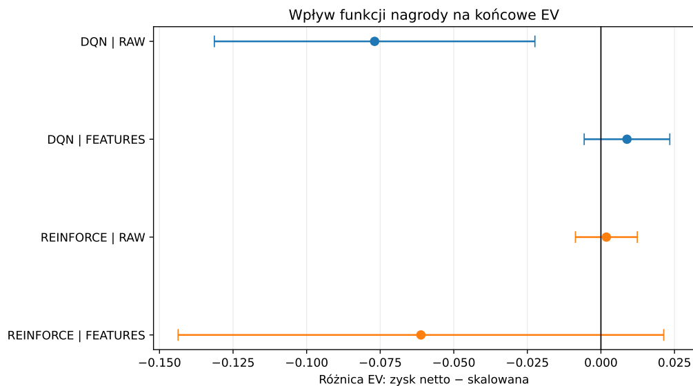
Rys. 7.3. Wpływ funkcji nagrody na końcowe EV. Punkty przedstawiają średnią różnicę EV_{\text{net}} - EV_{\text{scaled}} dla pięciu sparowanych seedów treningowych, a wąsy odpowiadają 95-procentowym przedziałom ufności.
