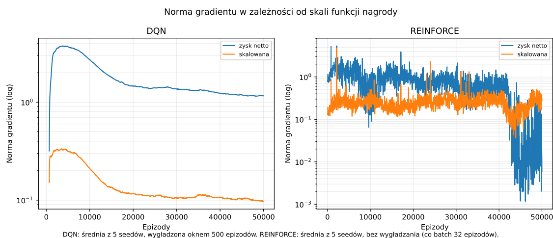
Rys. 7.8. Norma gradientu w zależności od skali funkcji nagrody dla konfiguracji wykorzystujących reprezentację FEATURES. Dla DQN przedstawiono średnią z pięciu seedów wygładzoną oknem 500 epizodów, natomiast dla REINFORCE średnią z pięciu seedów bez dodatkowego wygładzania. Oś pionowa ma skalę logarytmiczną.
