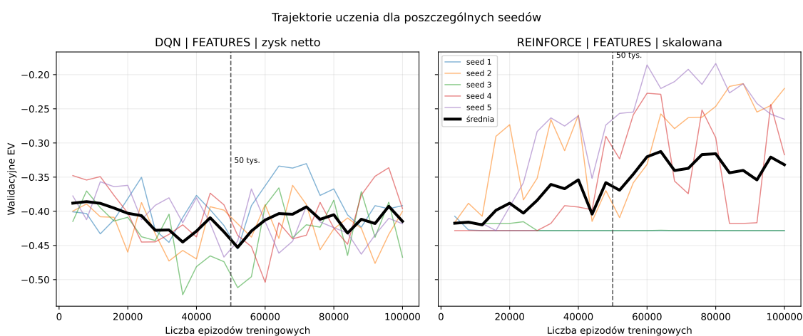
Rys. 7.6. Trajektorie walidacyjnego EV dla pięciu seedów wybranych konfiguracji DQN i REINFORCE podczas treningu do 100 000 epizodów. Linia pionowa oznacza podstawowy budżet 50 000 epizodów.
