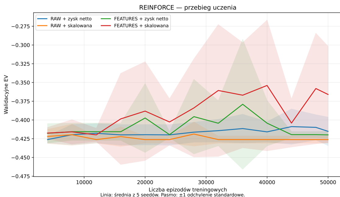
Rys. 7.5. Przebieg uczenia czterech konfiguracji REINFORCE. Linie przedstawiają średnie walidacyjne EV z pięciu seedów, a pasma jedno odchylenie standardowe między przebiegami treningowymi.
