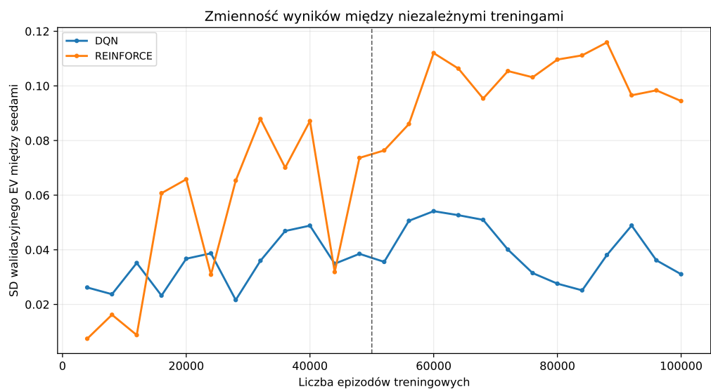
Rys. 7.10. Zmienność walidacyjnego EV między seedami podczas treningu
