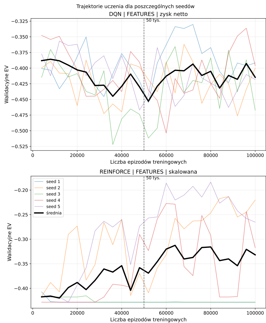
Rys. 7.9. Trajektorie walidacyjnego EV dla pięciu seedów wybranych konfiguracji DQN i REINFORCE
