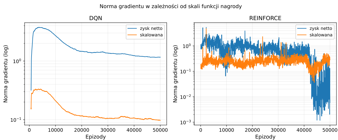
Rys. 7.11. Norma gradientu w zależności od skali funkcji nagrody
