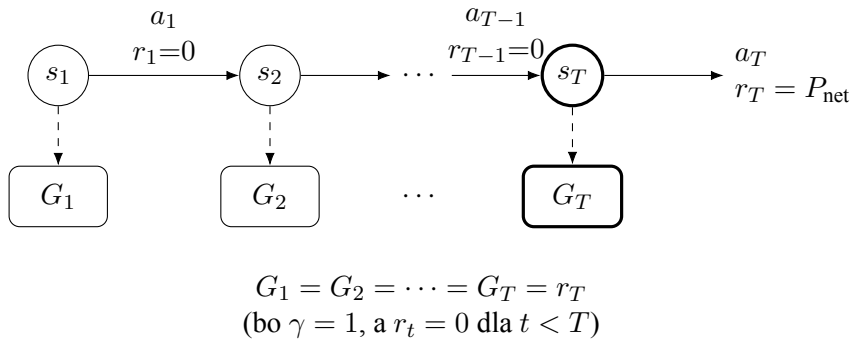
Rys. 5.7. Zwrot G_t w epizodzie REINFORCE
