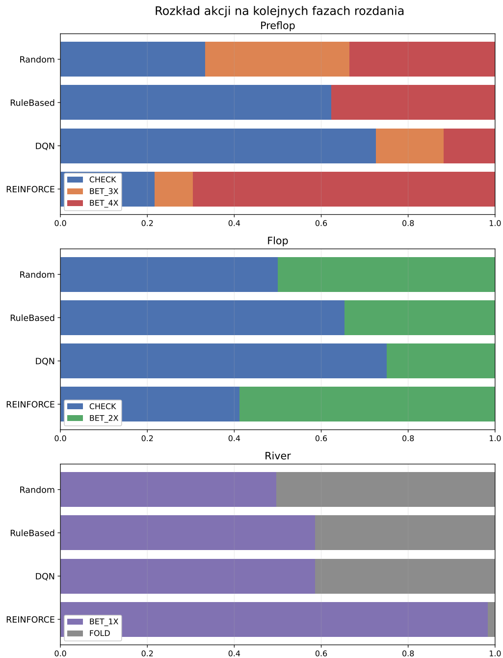
Rys. 7.13. Rozkład akcji na kolejnych fazach rozdania
