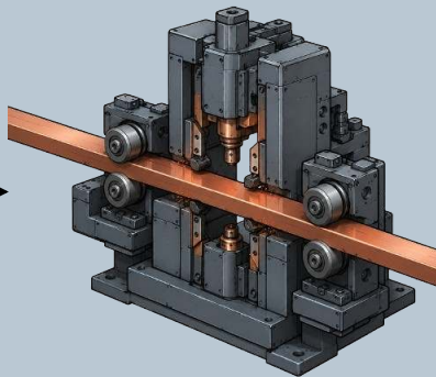
5. Remoção de rebarbas
