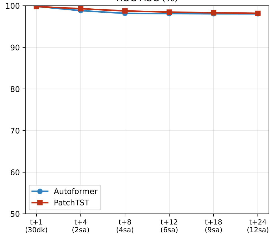
ROC-AUC (%)
