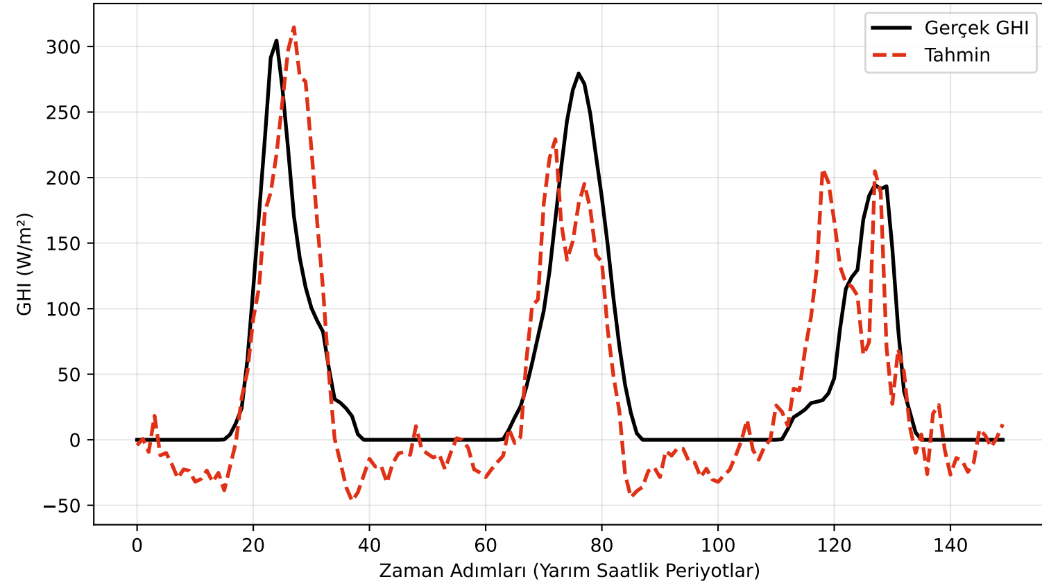
Hedef: 12 Saat Sonrası (t+24)
