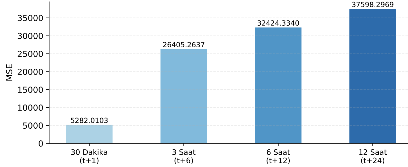
MSE
