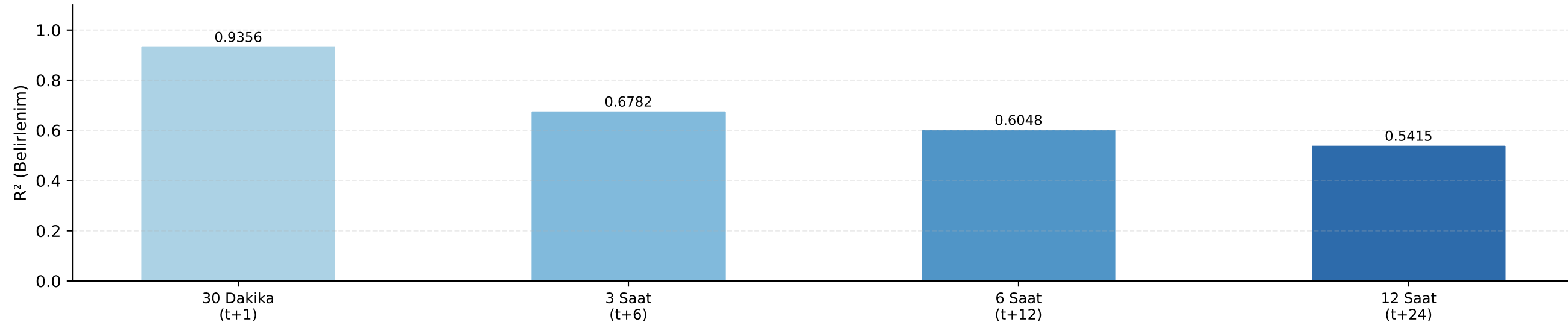
R 2 (Belirlenim)
