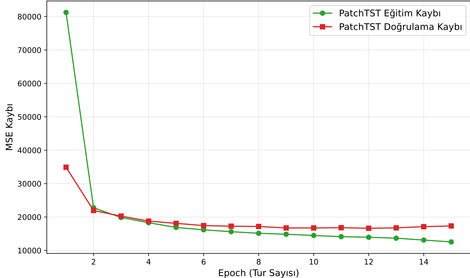
PatchTST Öğrenme Eğrisi (Learning Curve)
