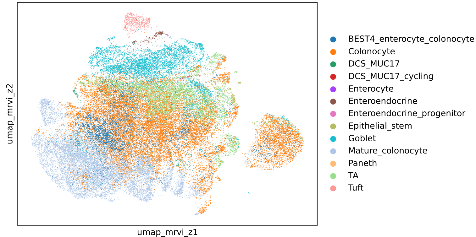
level_3_annot (mrvi_z)
