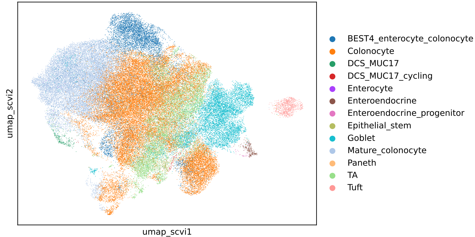
level_3_annot (scvi)
