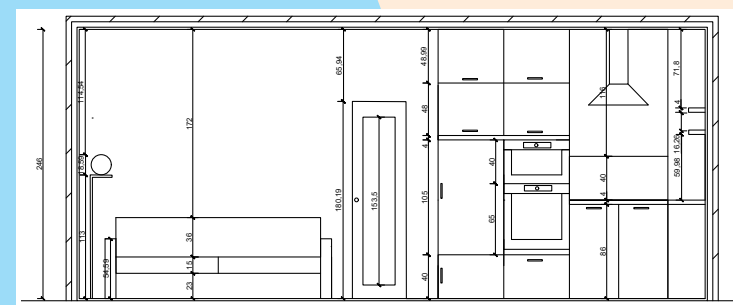
Coupes aménagées côté (autocad)
