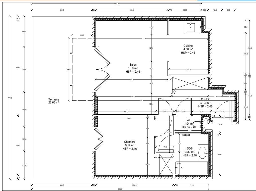
Plan EDE côté (autocad)
