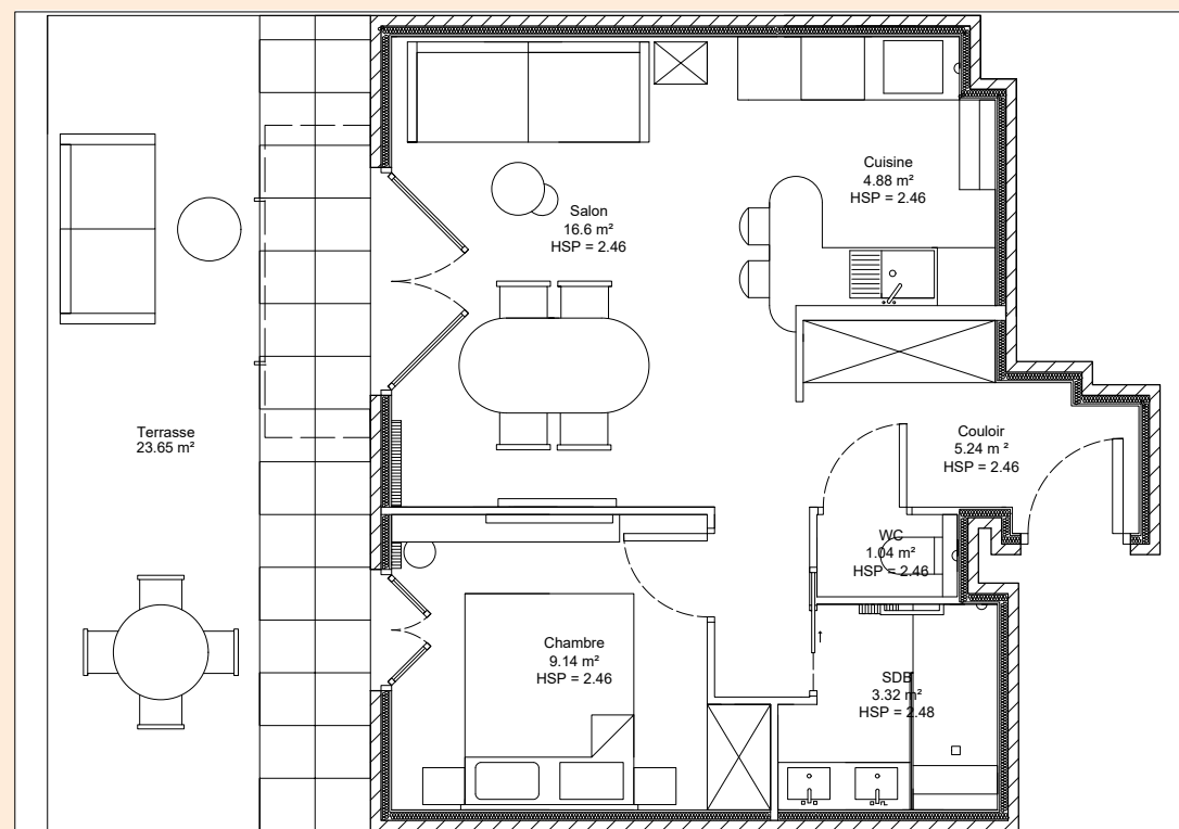
Plan aménagé (autocad)
