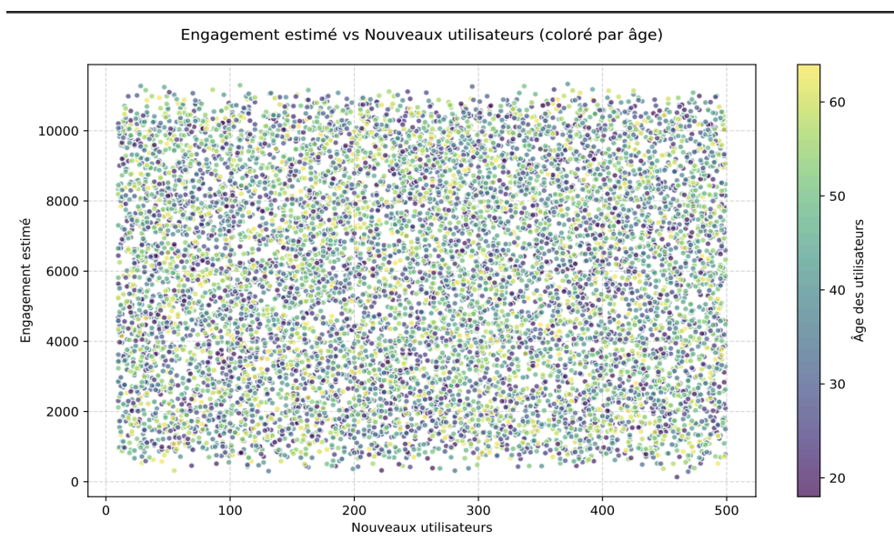
Figure1 Nuage de points représentant la corrélation entre les nouveaux utilisateurs et l'engagement estimé
